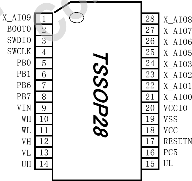
图表 3 管脚图
